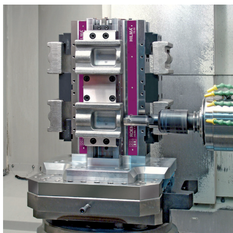
Turmspannsystem TS 125 mit 3.-Hand-Funktion
