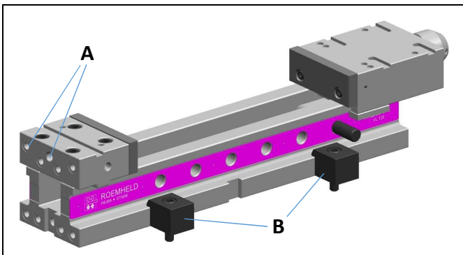
Abb. 2: Montagearten für Baureihe VL
