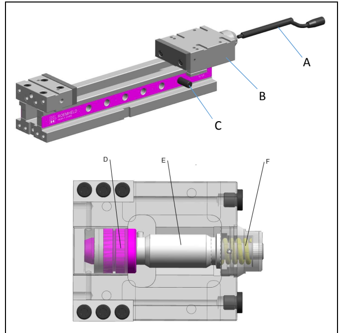
Abb. 1: Komponenten für Baureihe VL
