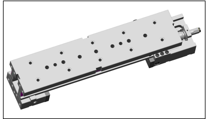
Abb. 3: Untersicht mit Befestigungs- und Positionsbohrungen
