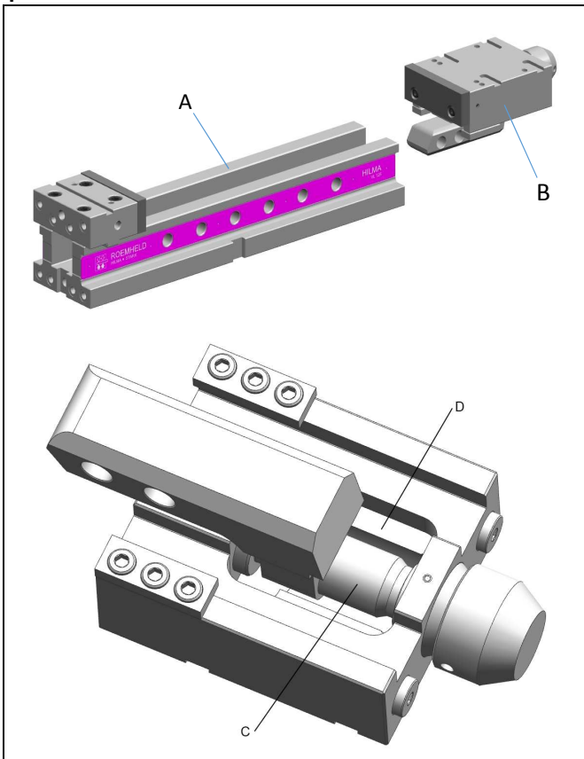
Abb. 8: Spannschlitten demontieren
