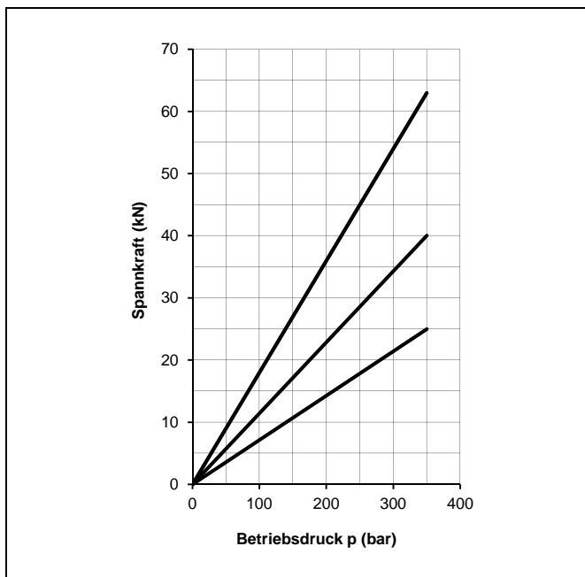
Abb. 9: Spannkraftverhältnisse
