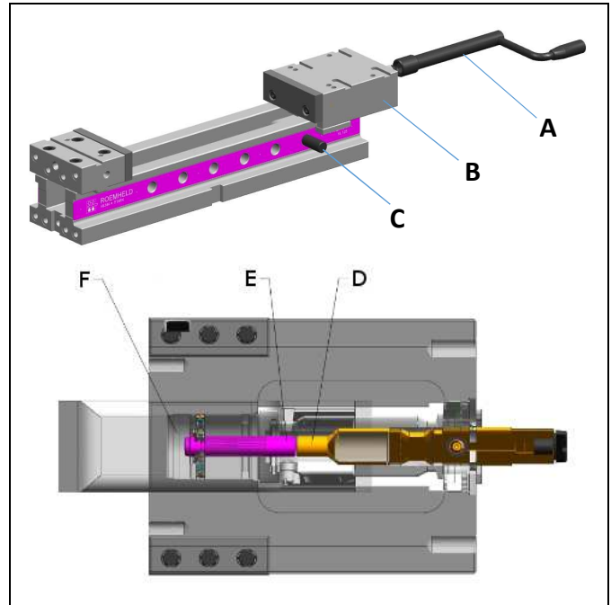
Abb. 1: Komponenten für Baureihe VL
