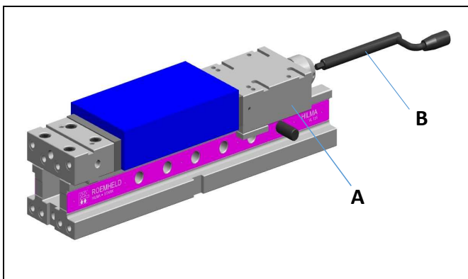
Abb. 6: Spannen und Lösen
