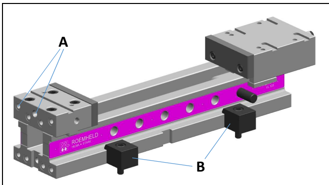
Abb. 2: Montagearten für Baureihe VL
