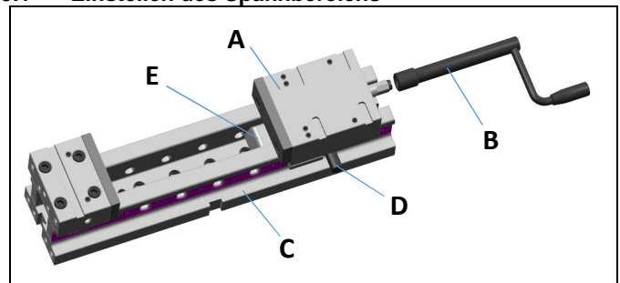
Abb. 4: Einstellen des Spannbereiches
