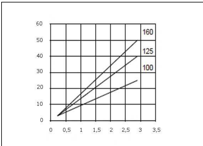
Abb. 11: Spannkraftverhältnisse
