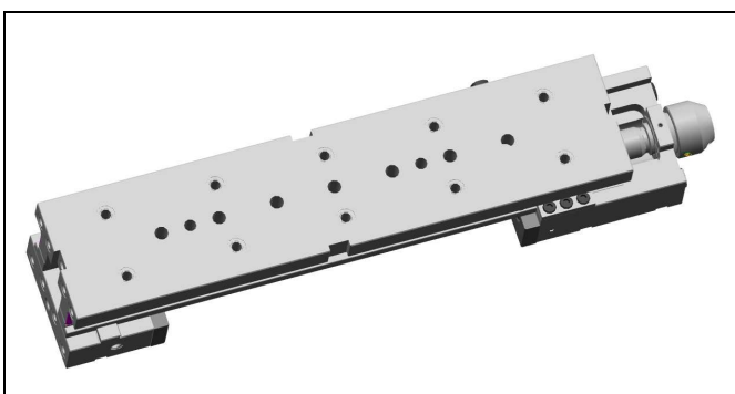
Abb. 3: Untersicht mit Befestigungs- und Positionsbohrungen
