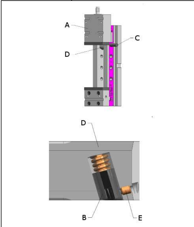
Abb. 7: Bremse für Spanschlitten BB 100 + 125
