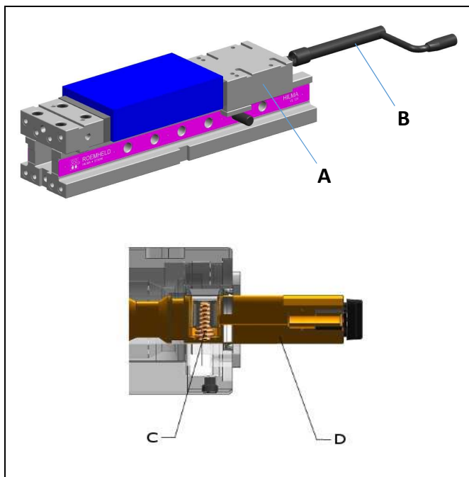
Abb. 5: Spannen und Lösen
