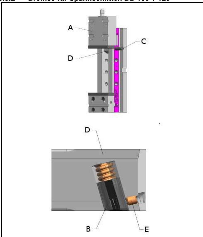
Abb. 6: Bremse für Spannschlitten BB 100 + 125
