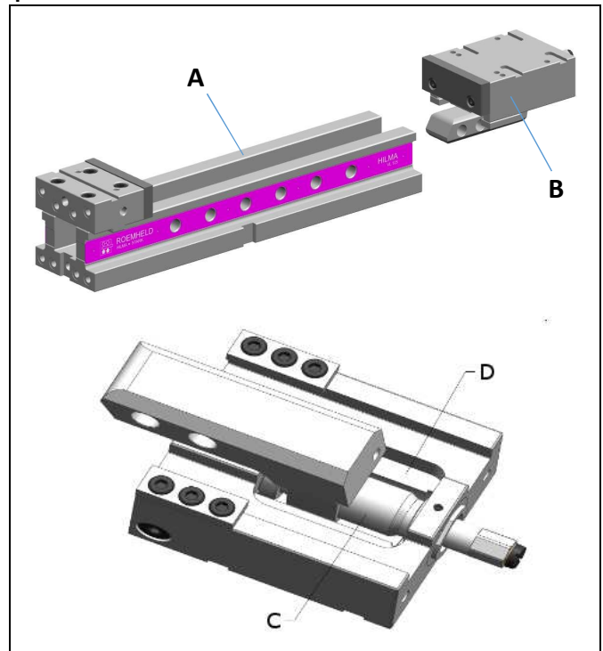
Abb. 8: Spannschlitten demontieren
