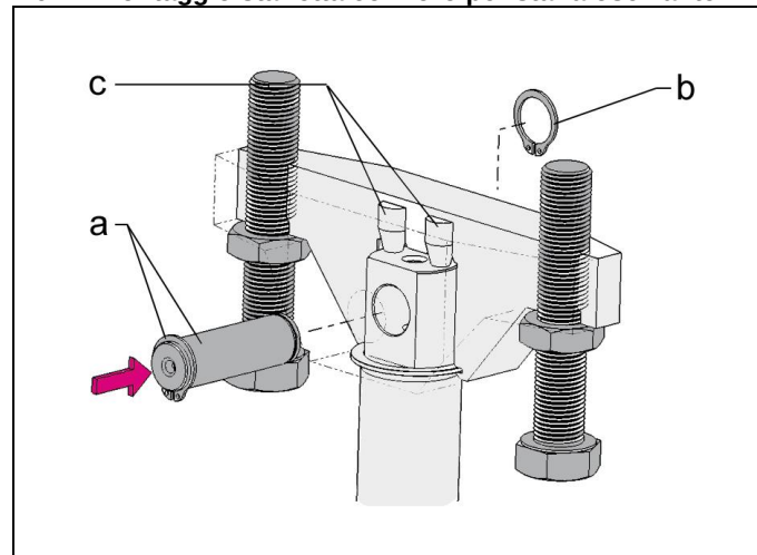
Fig. 6: Montaggio / smontaggio della staffetta oscillante
