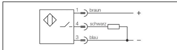
Fig. 10: Schema elettrico per il sensore magnetico pnp(+)
