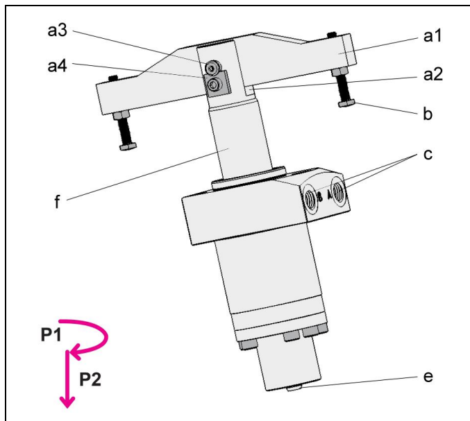
Fig. 2: Componenti, testa a forcella (max. 160 bar)
