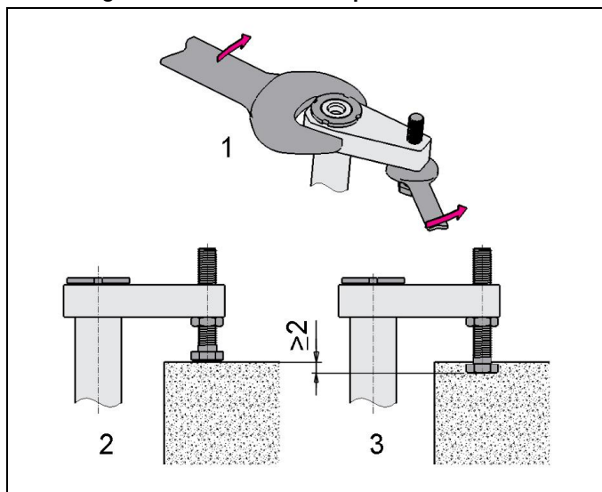
Fig. 8: Esempio di regolazione di una staffetta
