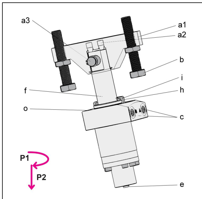
Fig. 1: Componenti, foro per staffa oscillante (max 500 bar)
