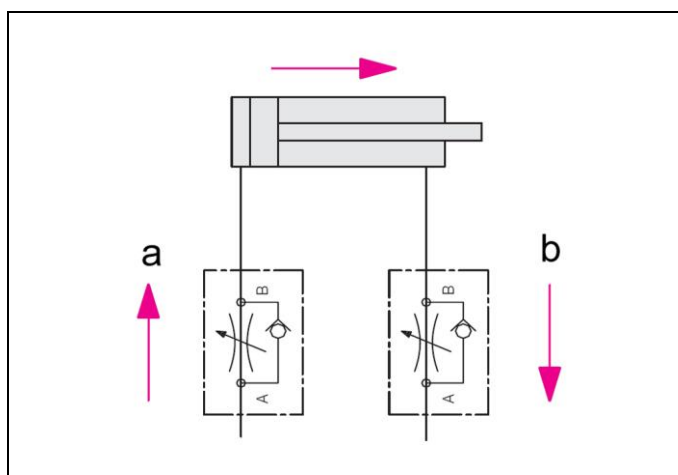
Fig. 4: Schema idraulico con valvole di ritenuta e strozzamento
