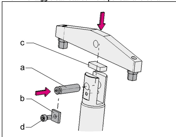
Fig. 7: Montaggio / smontaggio della staffetta oscillante
