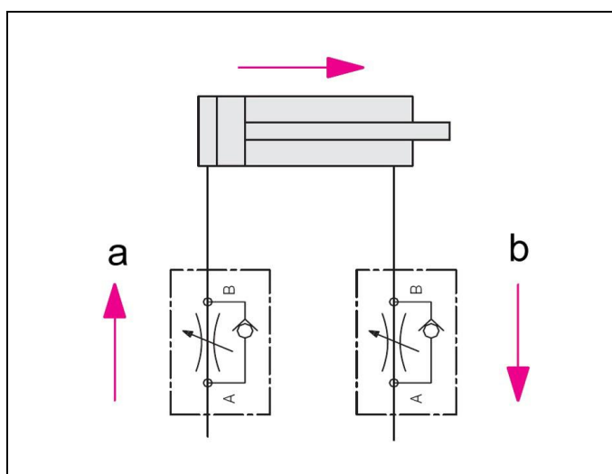
Fig. 8: Schéma hydraulique avec étrangleurs
