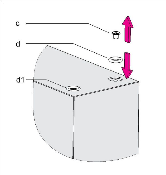
Fig. 9 : Exemple, préparation pour des connexions hydrauliques sans tuyauterie
