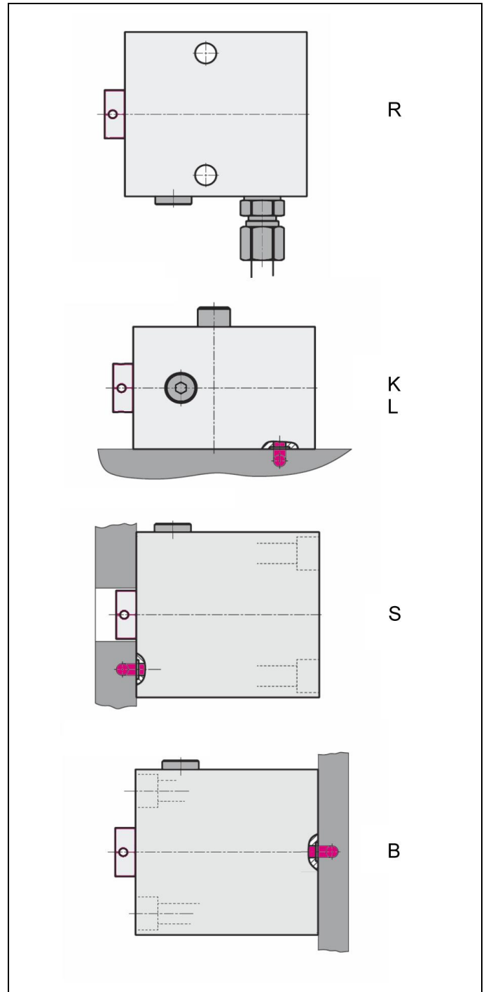
Fig. 4: Types de connexion des versions
