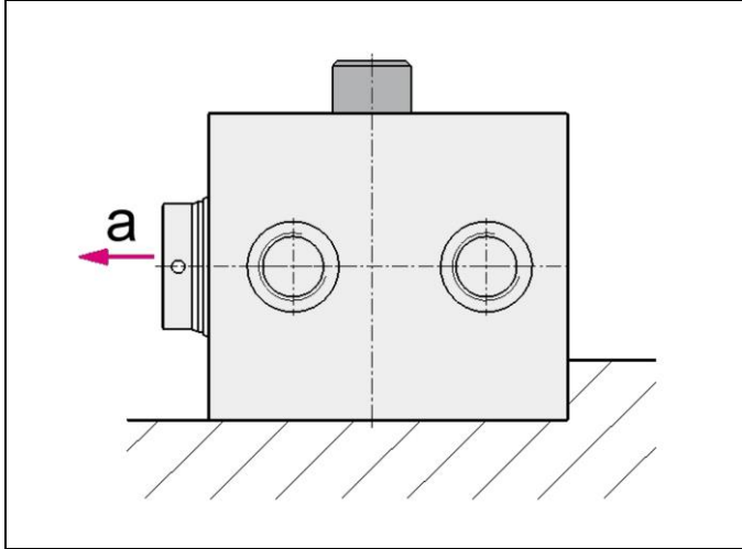
Fig. 5: Vérin-bloc appuyé
