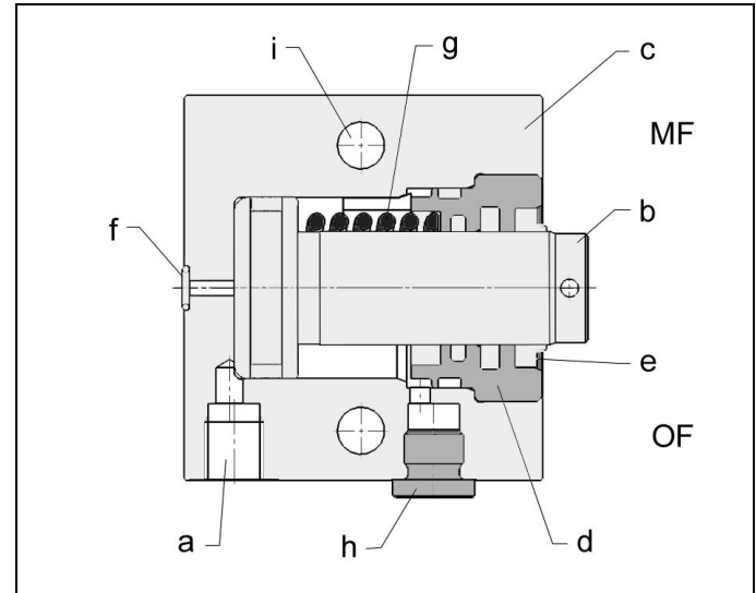
Fig. 1: Présentation de principe des composants
