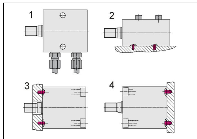
Fig. 3: Tipi di collegamento dell'alimentazione dell'olio idraulico
