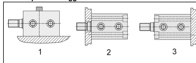
Fig. 2: Possibilità di fissaggio
