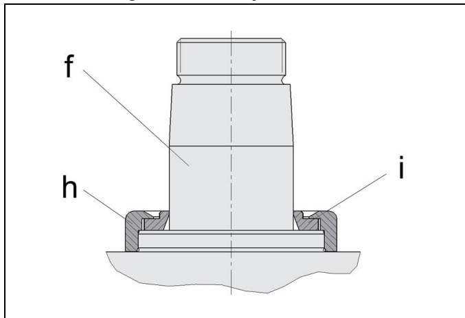
Bild 8: Metallavstrykare
