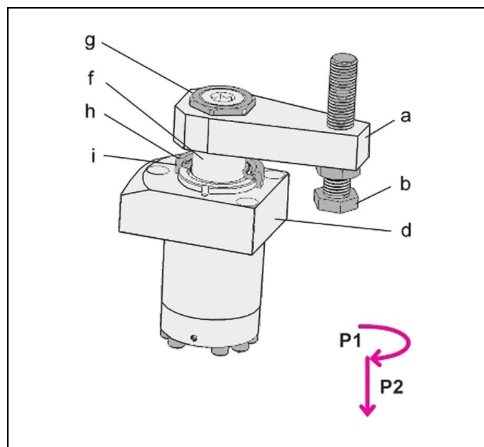
Bild 1: Komponenter
