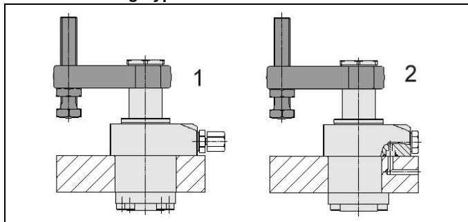
Bild 3: Monteringstyper
