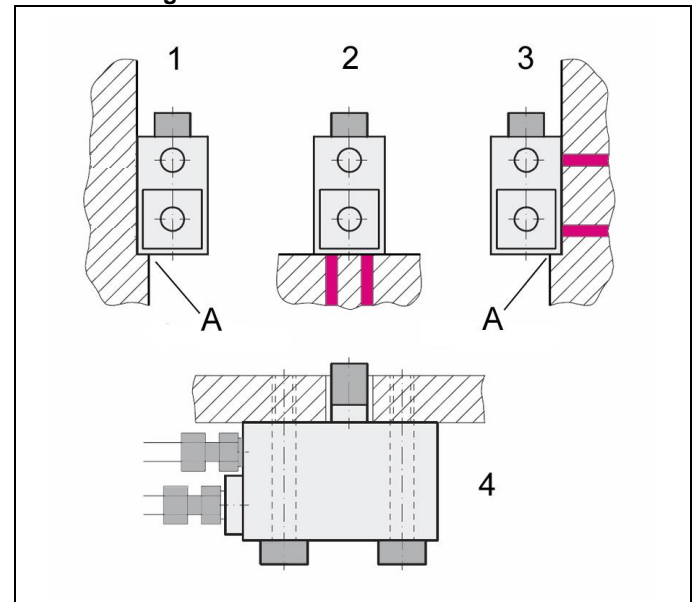
Abb. 2: Befestigungsart und Anschlussarten der Hydrauliközlufuhr
