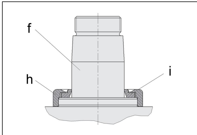
Fig. 8: Raschiatore metallico
