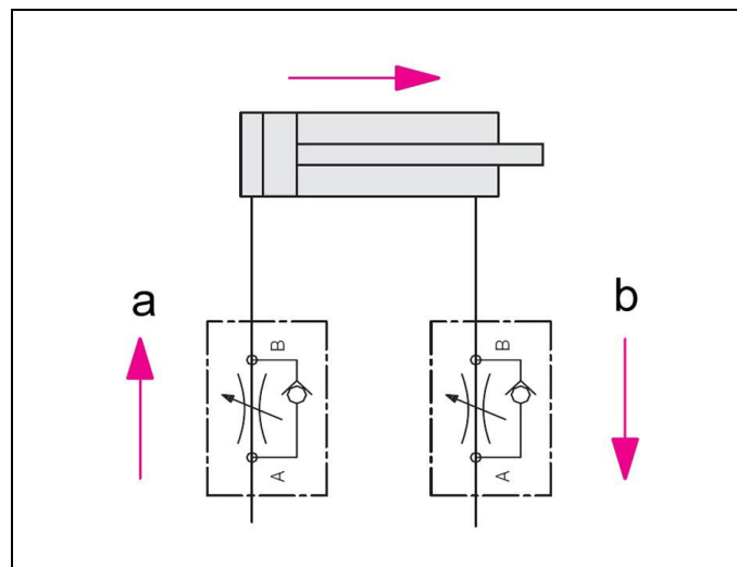
Slika 3: hidravlična shema z dušilnimi protipovratnimi ventili
