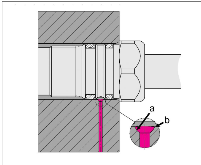
Slika 5: Vgradnja prek uvajalnega posnetega roba in prečne izvrtine
