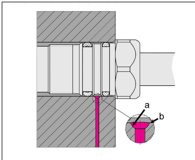
Fig. 5: Montaggio con smusso di inserimento e foro trasversale
