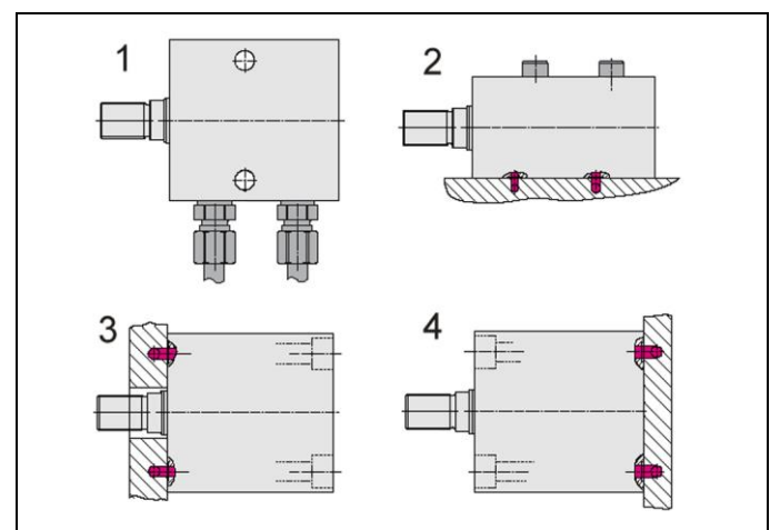
Abb. 3: Anschlussarten der Hydraulikölaufuhr
