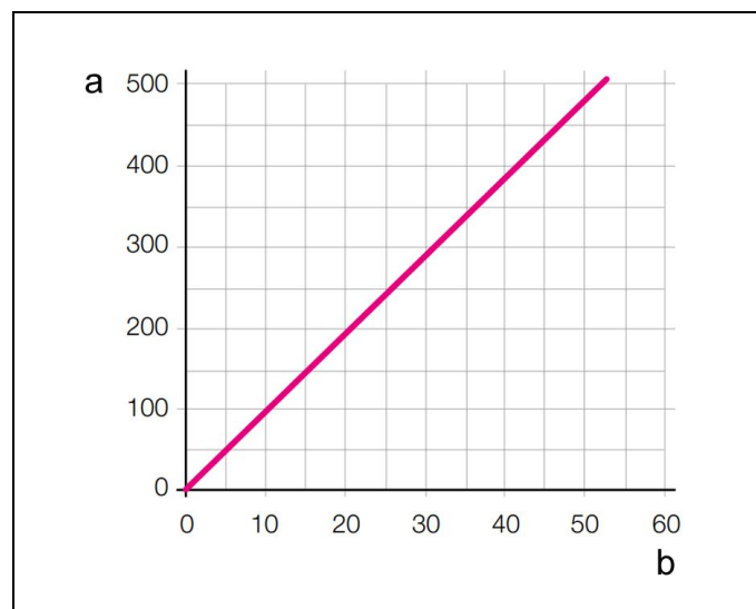
Fig. 4: Diagrama del par de apriete y la presión
