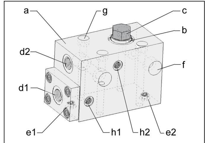
Fig. 1 : Composants
