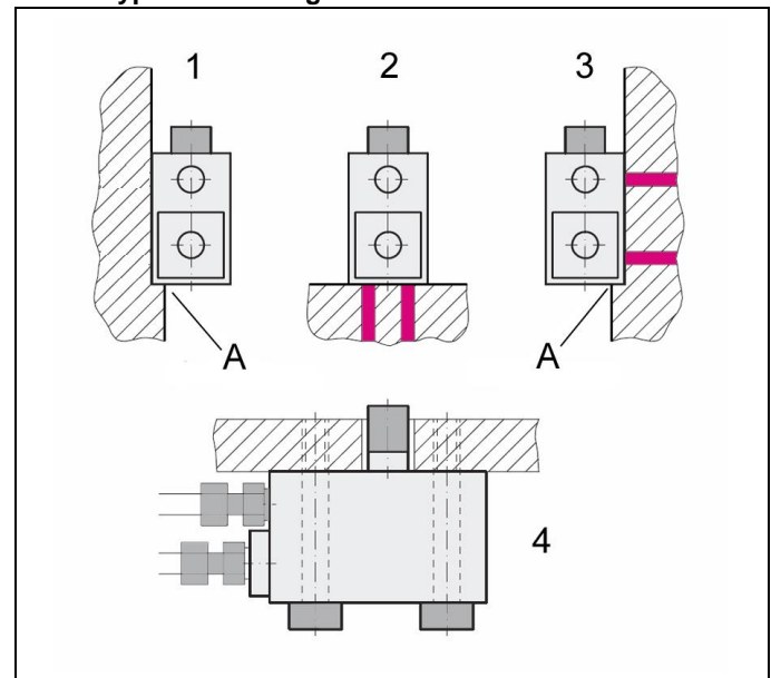
Fig. 2 : Types de fixation et de connexion de l'alimentation en huile hydraulique
