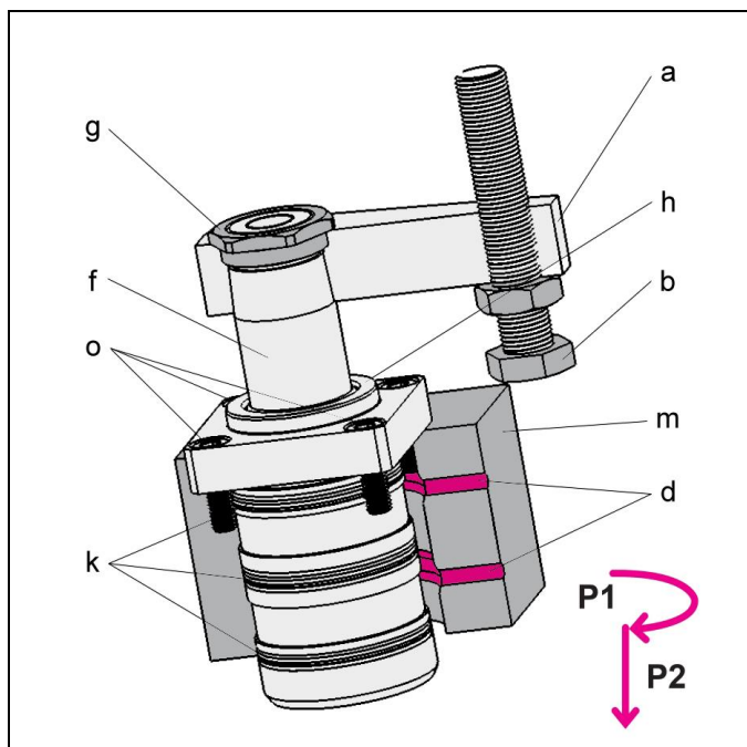
Abb. 1: Komponenten
