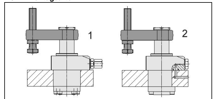
Abb. 3: Montagearten
