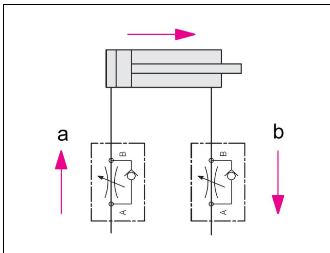
Fig. 2: Schéma hydraulique avec étrangleurs
