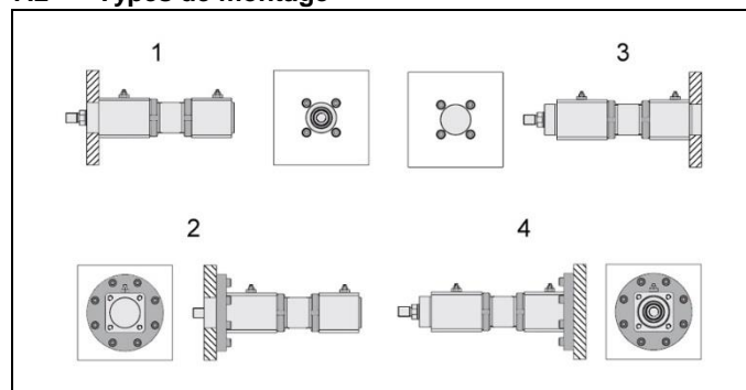
Fig. 2 : Possibilités de fixation
