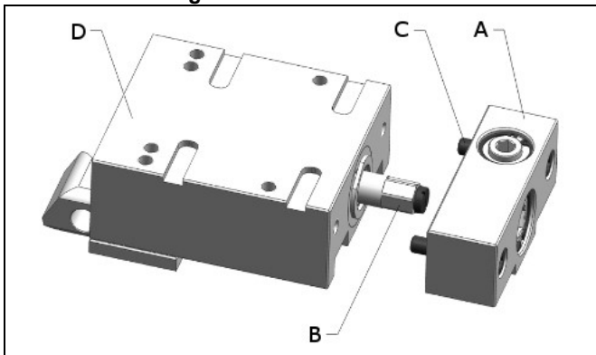
Fig. 7 : Renvoi d'angle
