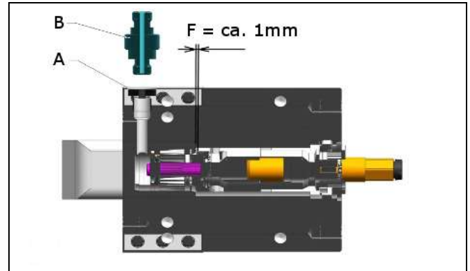
Fig. 9 : Remplissage de l'huile hydraulique
