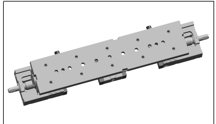
Fig. 3 : Vue de dessous avec alésages de fixation et de positionnement
