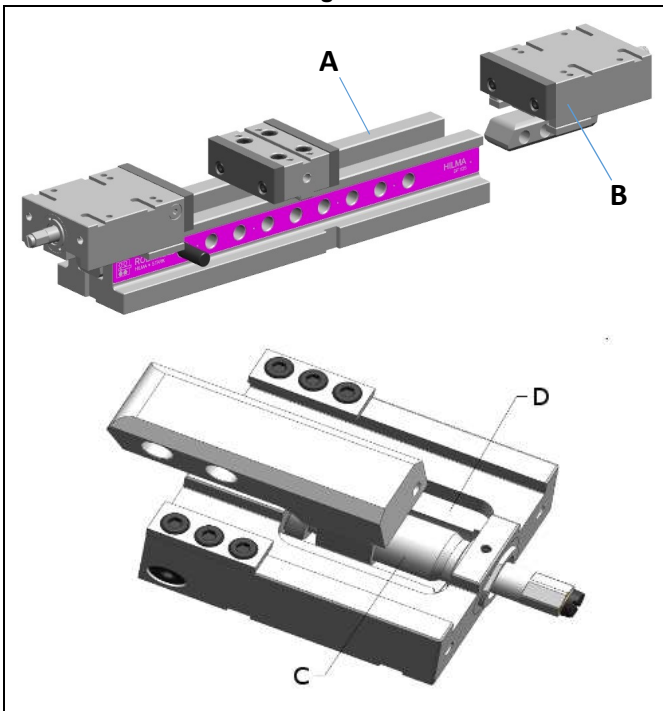
Fig. 8 : Démontez le chariot de serrage
