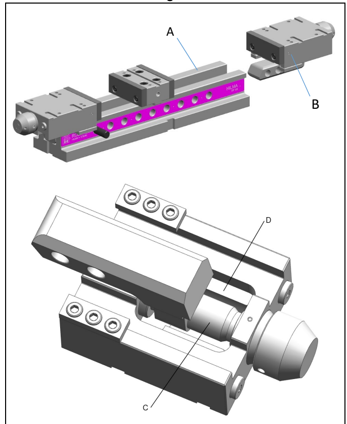
Fig. 8 : Démontez le chariot de serrage
