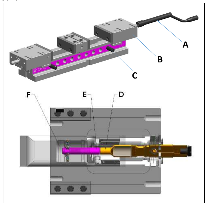
Fig. 1 : Composants pour la série DF
