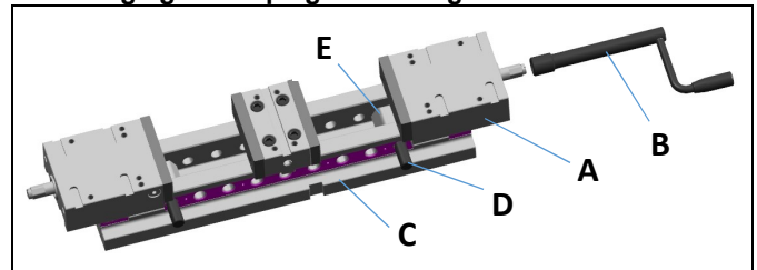
Fig. 4 : Réglage de la plage de serrage
