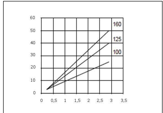
Fig. 11 : Rapports de force de serrage
