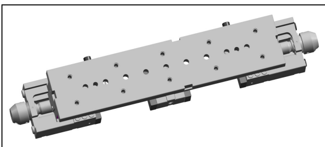
Fig. 3 : Vue de dessous avec alésages de fixation et de positionnement
