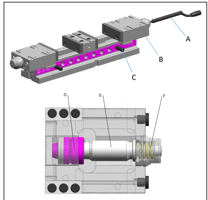
Fig. 1 : Composants pour la série DF
