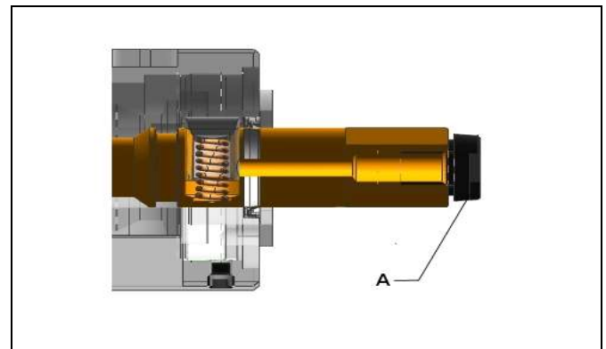
Fig. 10 : Lubrification du cran d'arrêt
