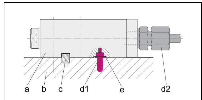
Fig. 2 : Composants
