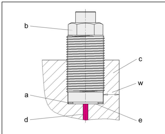
Fig. 6: Montage du joint axial sur la surface plane
