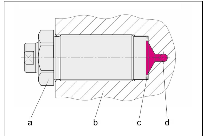
Fig. 1 : Composants
