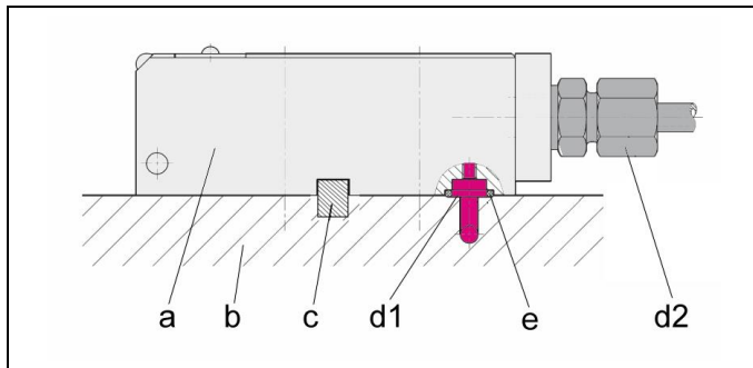
Fig. 3 : Composants
