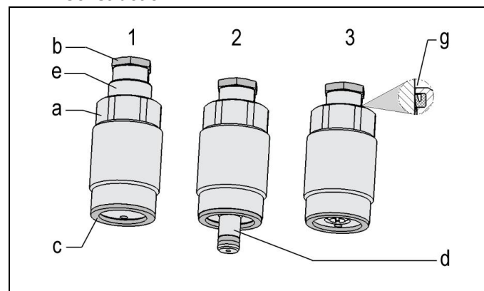
Fig. 1 : Composants
