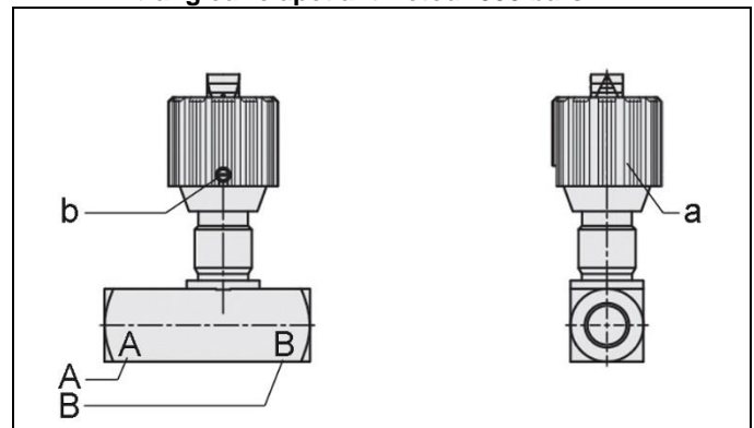
Fig. 2 : Étrangleur clapet anti-retour 350 bars
