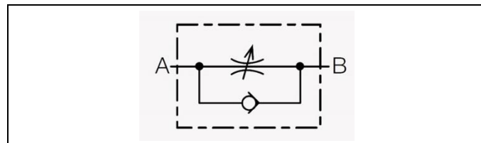
Fig. 5 : Étrangleur clapet anti-retour 350 bars
