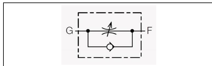
Fig. 6 : Étrangleur clapet anti-retour 500 bars
