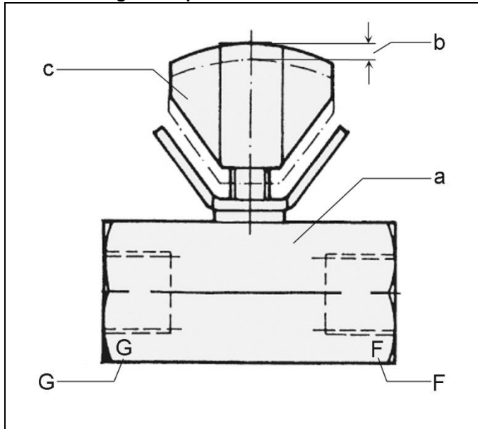
Fig. 3 : Étrangleur clapet anti-retour 500 bars
