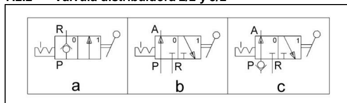
Fig. 2: Representación en el esquema hidráulico
