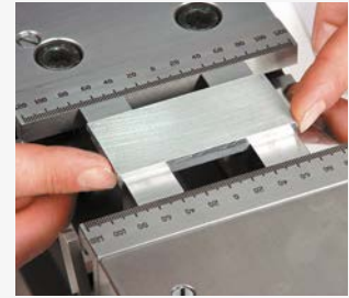
3. Insérer l'ébauche de pièce à usiner à vue d'œil au milieu et serrer.
