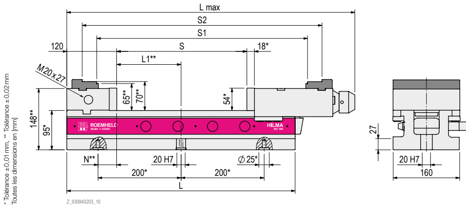
Figure : 930840203 Étendue de livraison standard : Étau de machine, manivelle et mors de serrage incl.
