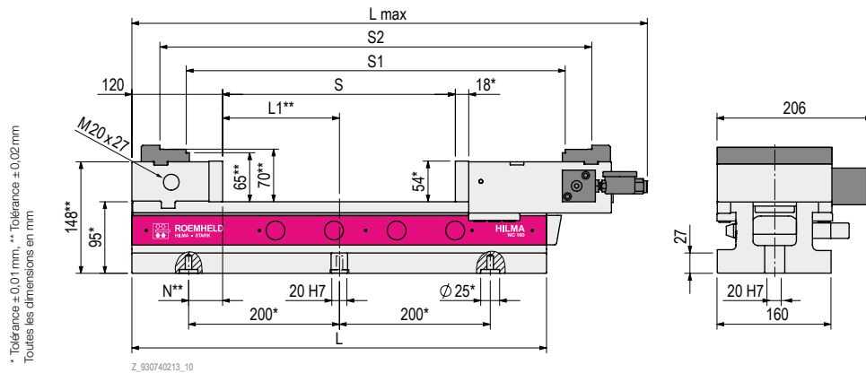
Figure : 930740203 Étendue de livraison standard : Étau de machine, manivelle et mors de serrage incl.
