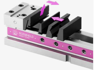
Relever le mors amovible QIS jusqu'à l'extrémité de la gorge et le basculer
