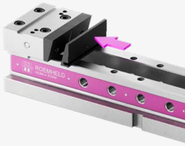
Guider parallèlement le mors amovible QIS & le placer avec le goujon
