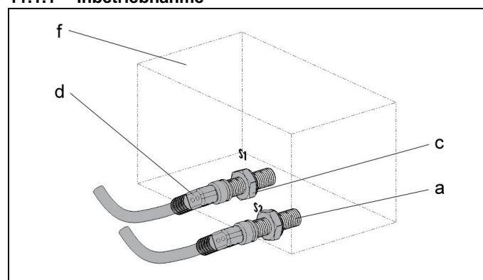
Abb. 6: Komponenten (Prinzip Einbau in einer Spannpratze)
