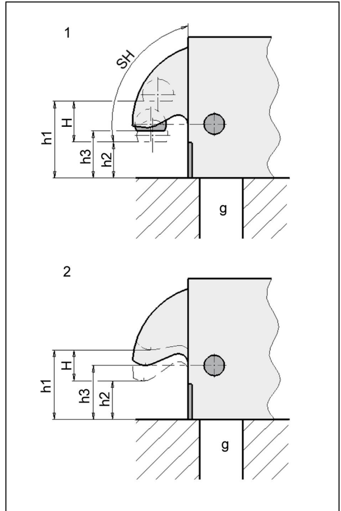
Abb. 2: Ausführungen der Spannhebel
