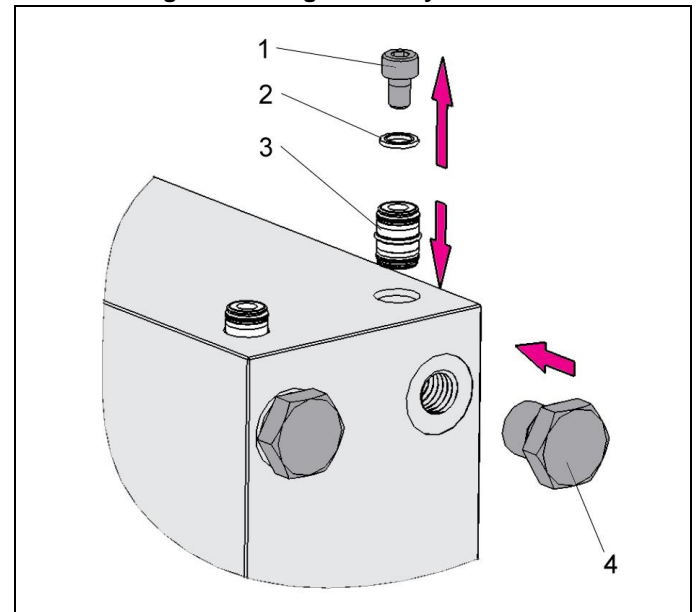
Abb. 5: Beispiel der Vorbereitung für leitungslose Hydraulikan- schlüsse mittels Steckverbindung
