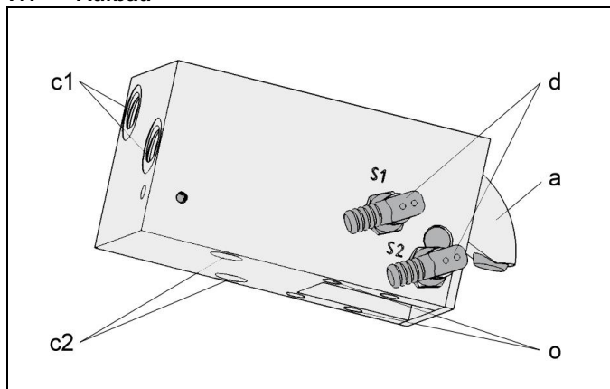
Abb. 1: Komponenten
