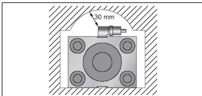
Fig. 9: Distancia mínima de los sensores a los protectores, etc.
