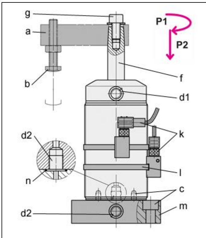
Fig. 1: Componentes
