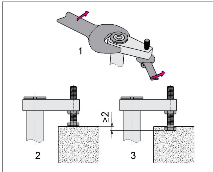
Fig. 5: Regulación de la brida de sujeción - ejemplo
