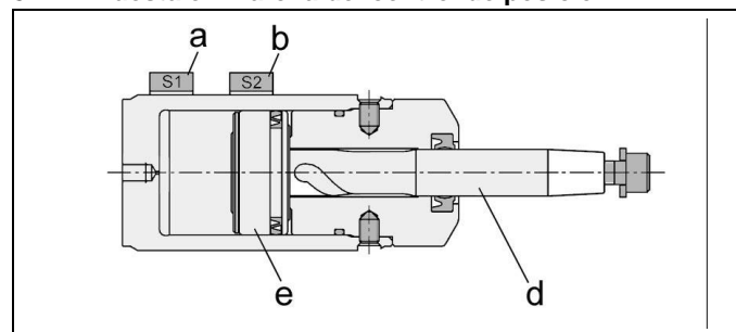
Fig. 6: Construcción
