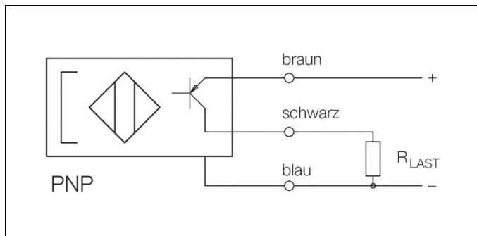
Fig. 8: Esquema eléctrico para PNP (+) sensor magnético
