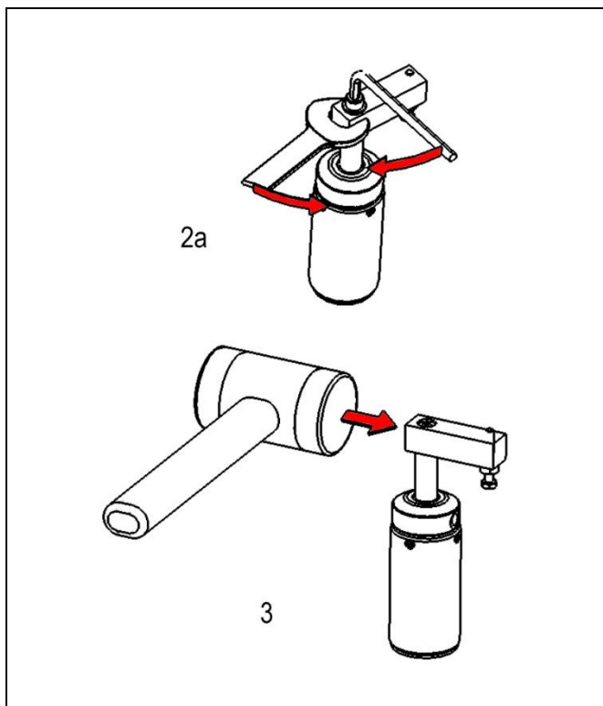
Fig. 4: Montaje / desmontaje - ejemplo
