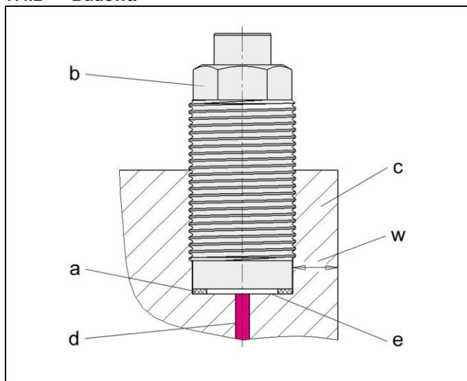
Ilustracja 4: Montaż uszczelnienia osiowego na płaskiej powierzchni obróbkowej
