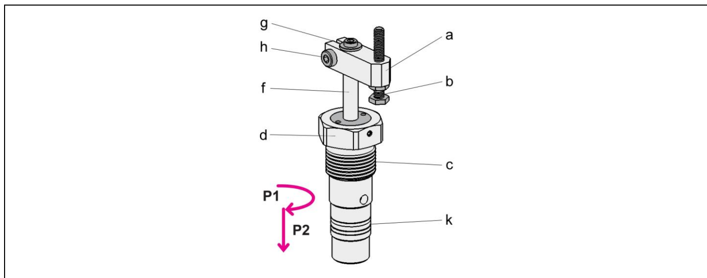
Fig. 2: Componenti
