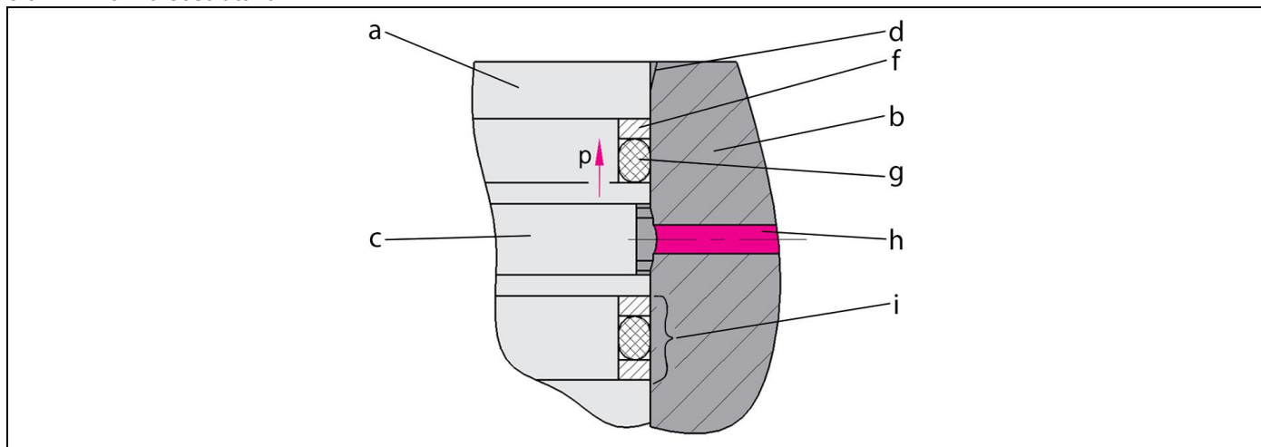
Fig. 5: Componenti
