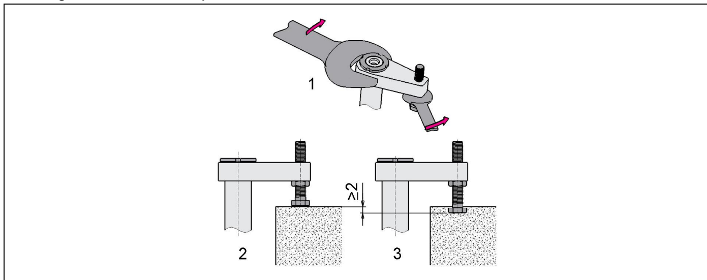
Fig. 8: Esempio di regolazione di una staffetta
