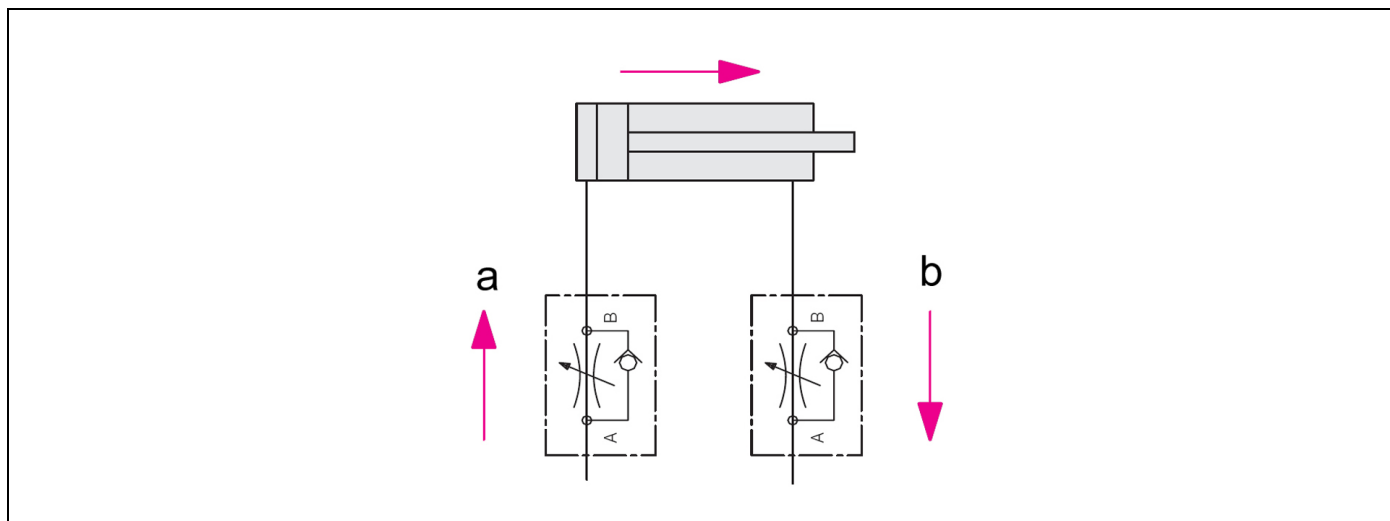
Fig. 4: Schema idraulico con valvole di ritenuta e strozzamento
