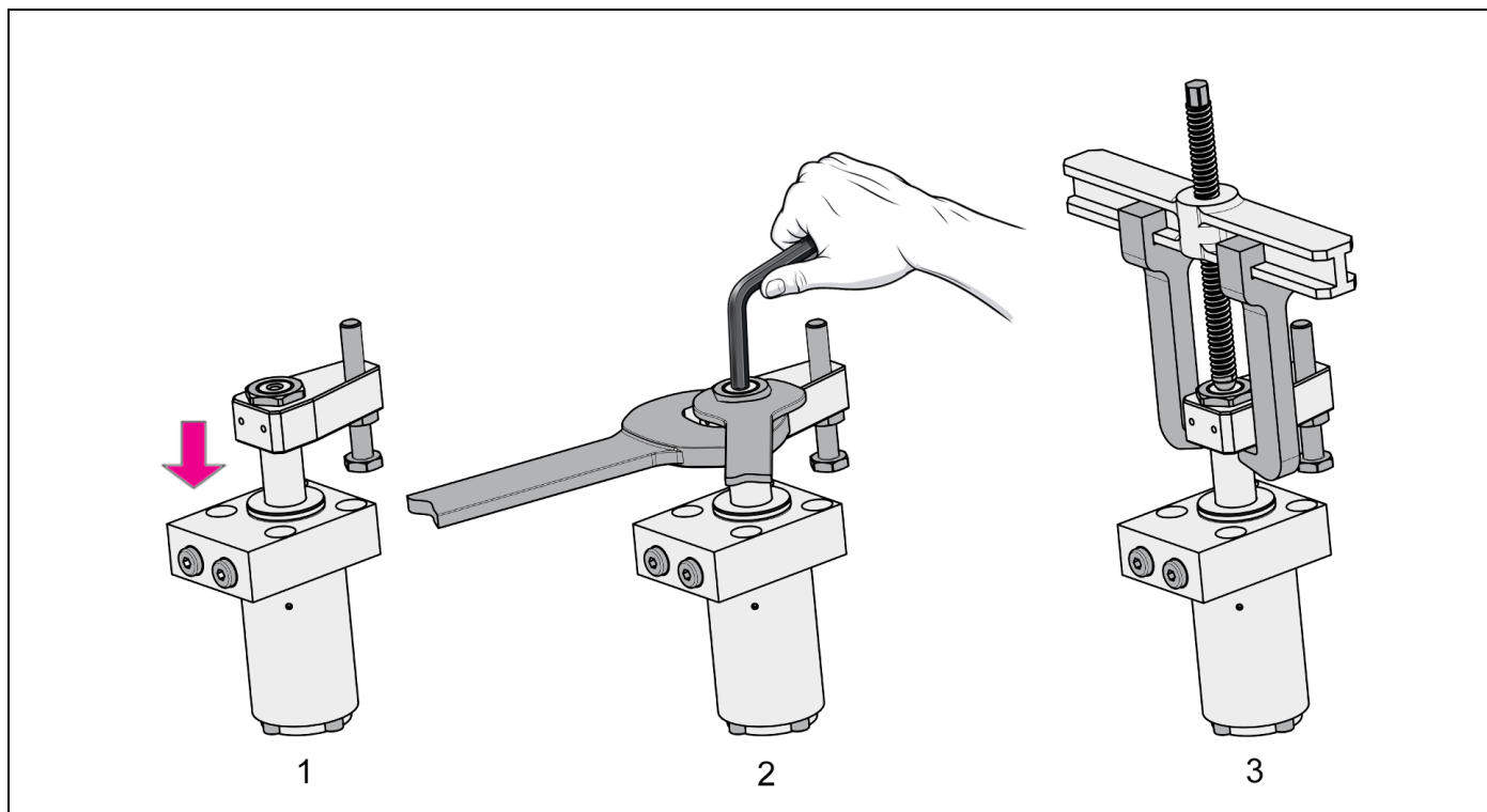
Fig. 7: Esempio di montaggio e smontaggio
