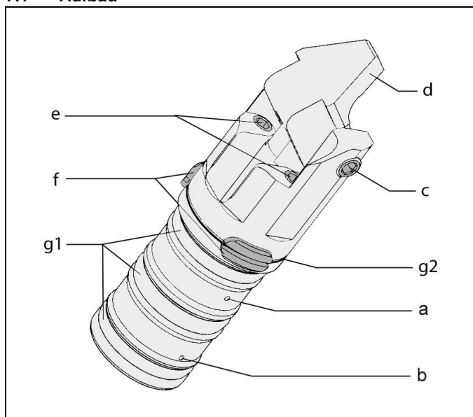
Abb. 1: Komponenten
