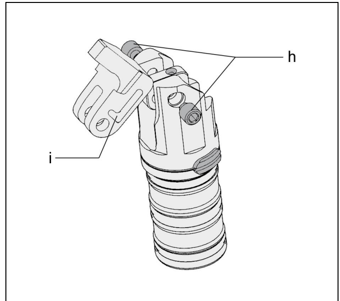
Abb. 7: Kompaktspanner
