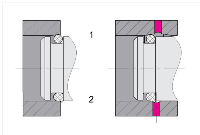
Abb. 6: Einbau über Einführungsfasen und Querbohrung
