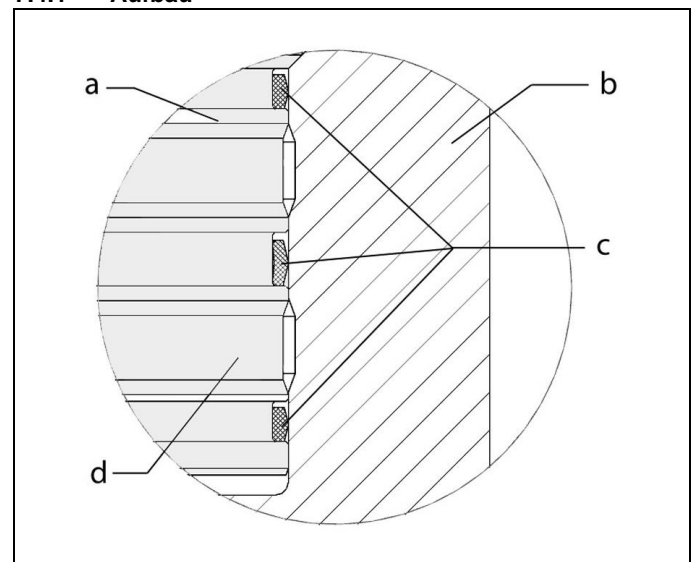
Abb. 5: Komponenten
