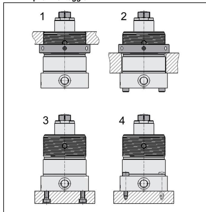
Fig. 2: Possibilità di fissaggio
