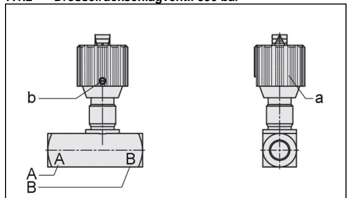
Abb. 2: Drosselückschlagventil 350 bar
