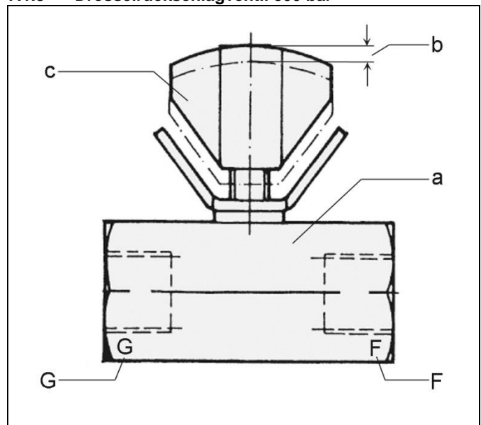
Abb. 3: Drosselückschlagventil 500 bar
