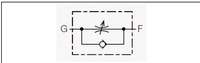
Abb. 6: Drosselrückschlagventil 500 bar
