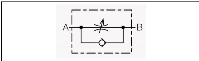
Abb. 5: Drosselrückschlagventil 350 bar
