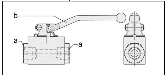
Abb. 1: Hochdruck-Absperrventil
