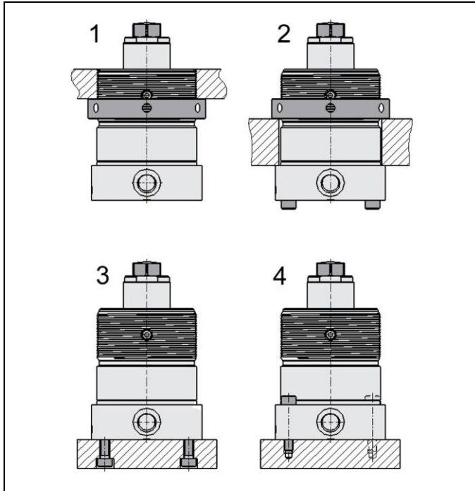
Fig. 2: Possibilités de fixation
