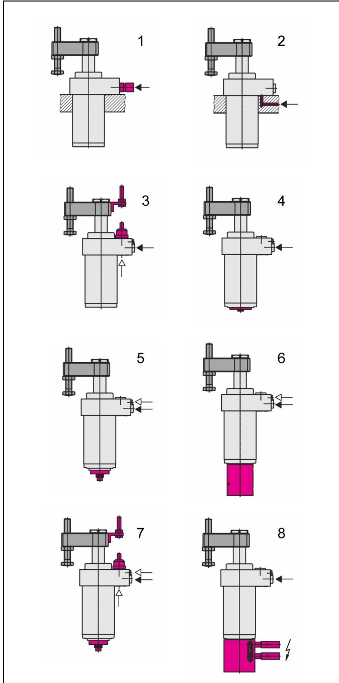
Abb. 3: Einbau- und Anschlussmöglichkeiten
