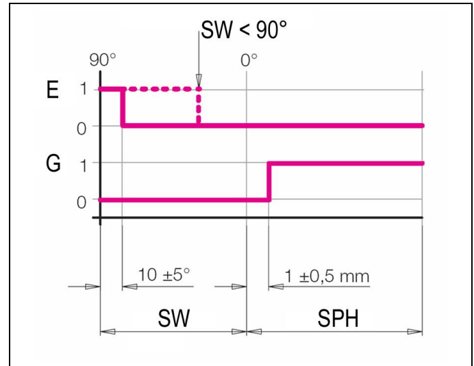
Abb. 14: Funktionsdiagramm
