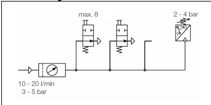
Abb. 15: Schematische Darstellung der Abfrage durch Druckschalter
