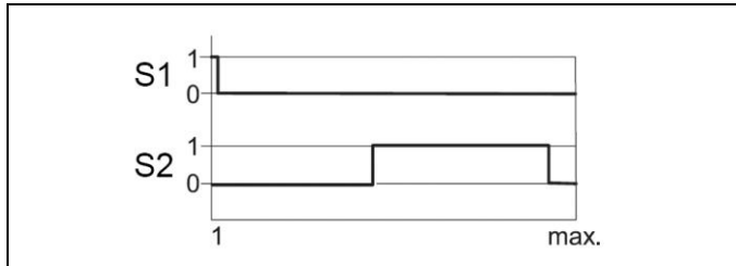
Abb. 12: Signalverlauf Entspannvorgang
