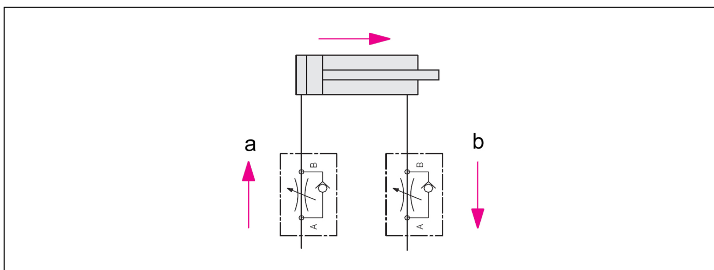
Fig. 2: Schéma hydraulique avec étrangleurs
