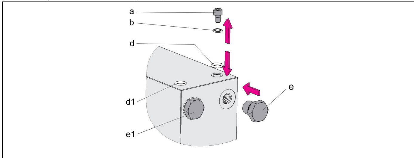
Fig. 3 : Exemple, préparation pour des connexions hydrauliques sans tuyauterie
