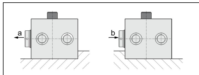
Fig. 2: Cilindro a basetta con appoggio
