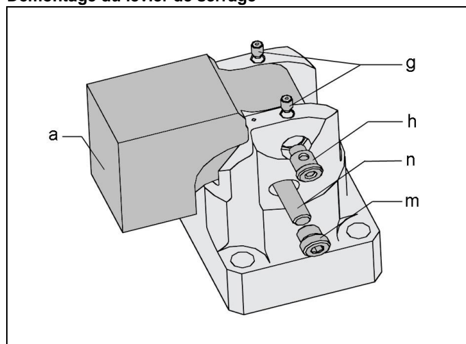
Fig. 4 : Démontage / montage du levier de serrage
