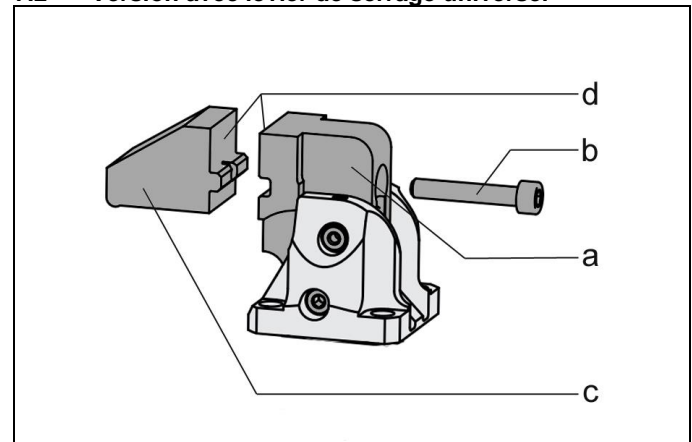
Fig. 2 : Composants
