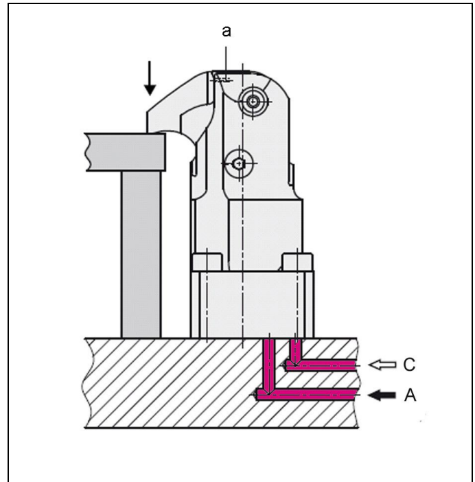
Fig. 6 : Contrôle de serrage
