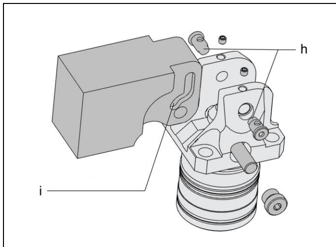
Fig. 13 : Brides compactes
