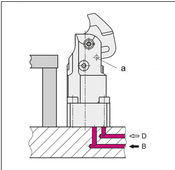
Fig. 9 : Contrôle de serrage
