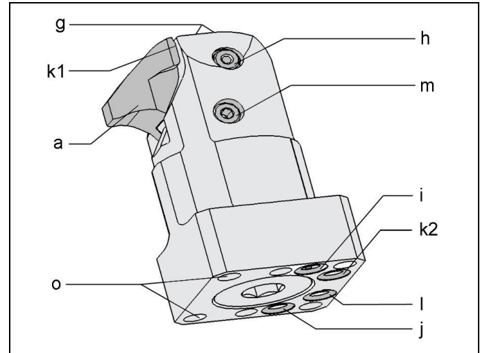
Fig. 1 : Composants
