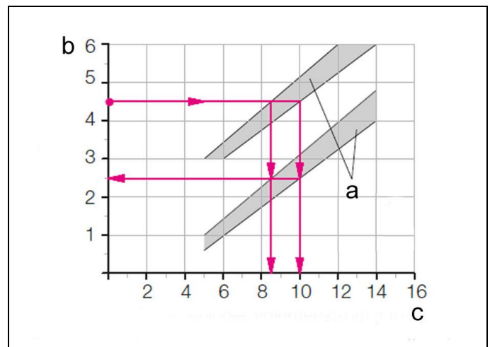
Fig. 11 : Contrôle de serrage
