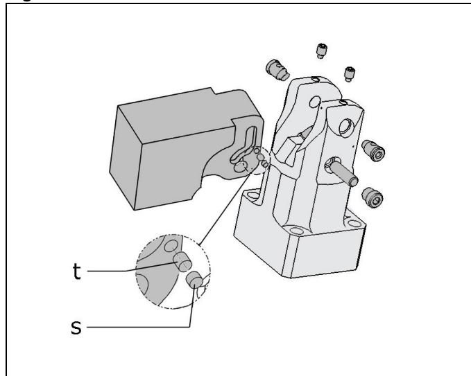
Fig. 5 : Démontage / montage du levier de serrage
