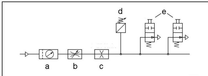
Fig. 12 : Schéma
