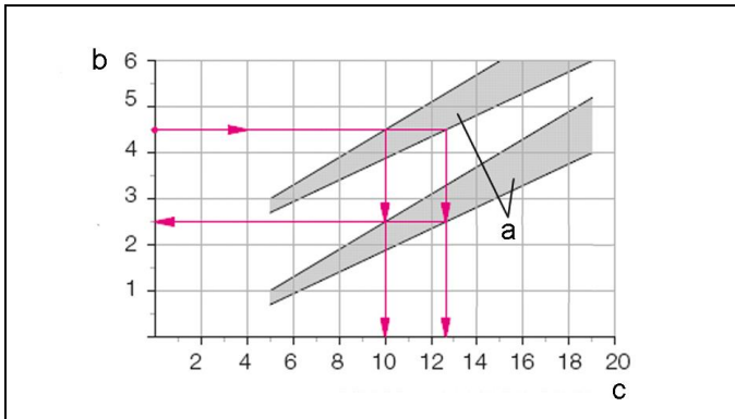
Fig. 8 : Contrôle de serrage
