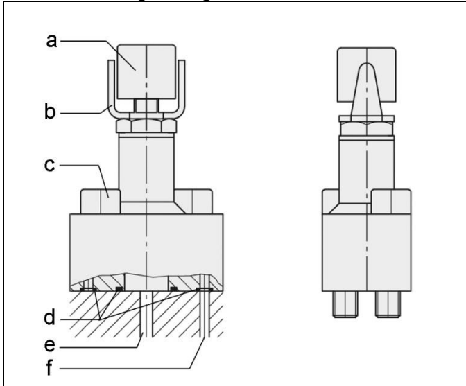
Abb. 2: Flanschanschluss
