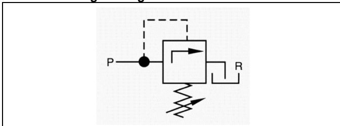
Abb. 3: Darstellung im Hydraulikplan
