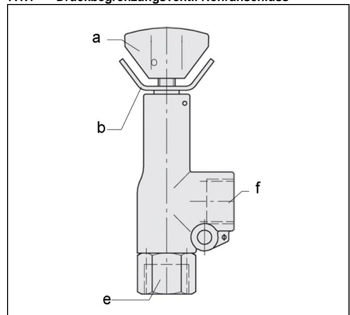
Abb. 1: Druckbegrenzungsventil Rohranschluss
