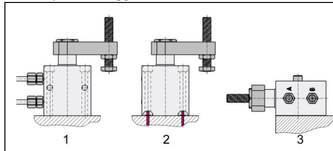
Fig. 3: Tipi di montaggio
