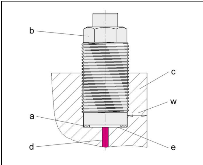
Abb. 6: Einbau der Axialdichtung auf Planfläche
