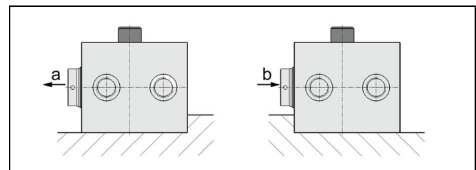
Abb. 2: Blockzylinder abgestützt
