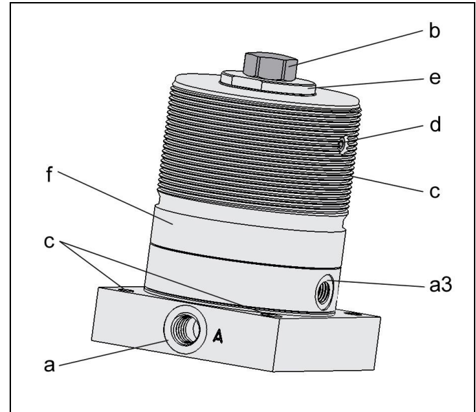
Fig. 1 : Composants
