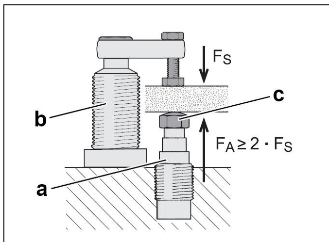
Fig. 3: Principio, flujo de fuerzas durante el apoyo
