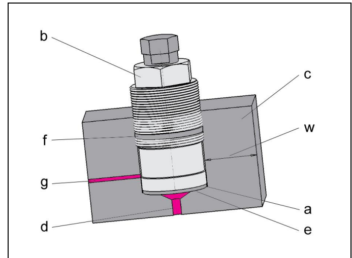
Fig. 4: Instalación de la junta axial en la superficie plana
