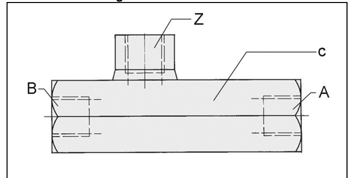
Abb. 1: Rohrgewindeanschluss
