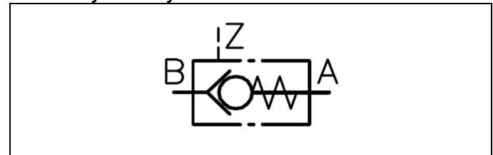
Abb. 2: Darstellung im Hydraulikplan
