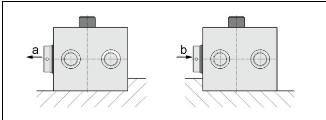
Abb. 3: Blockzylinder abgestützt
