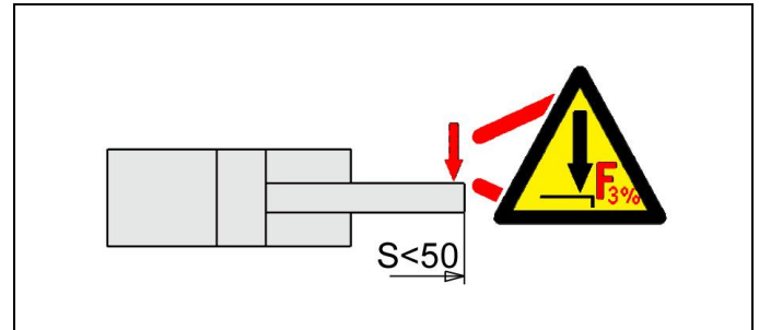
Abb. 5: Querkräfte einleiten
