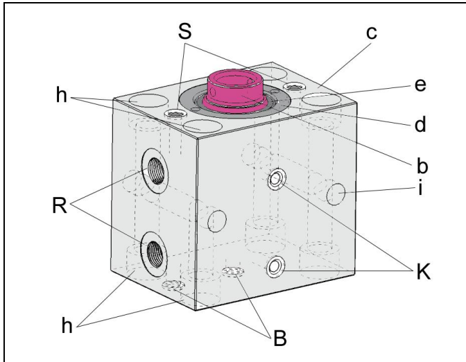
Abb. 1: Prinzipdarstellung der Komponenten und Anschlüsse
