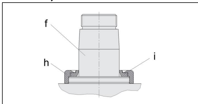
Fig. 8: Rascador metálico
