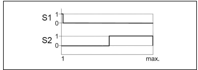
Fig. 11: Curva del señal - bloqueo
