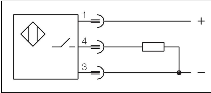
Fig. 9: Esquema eléctrico para pnp(+) sensor magnético
