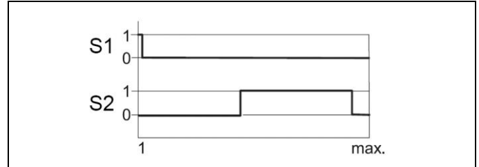
Fig. 12: Curva del señal - desbloqueo
