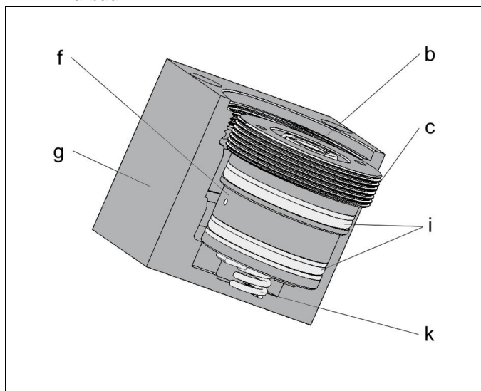
Abb. 1: Komponenten
