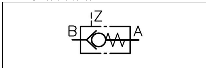
Fig. 2: Rappresentazione nello schema idraulico
