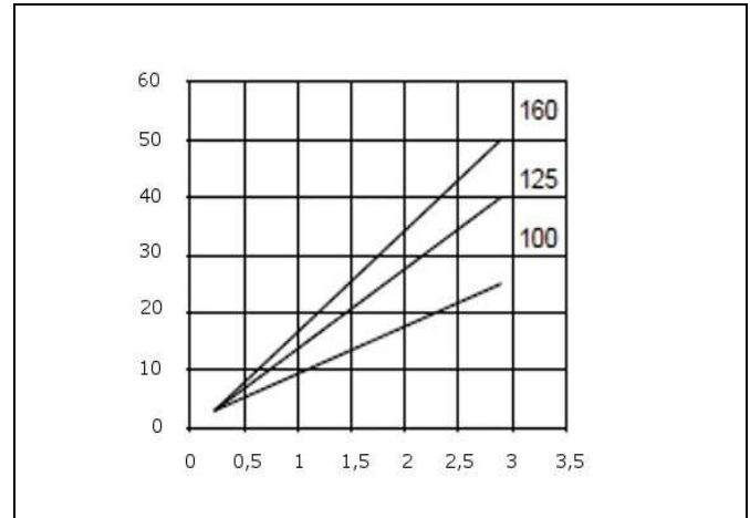
Abb. 11: Spannkraftverhältnisse
