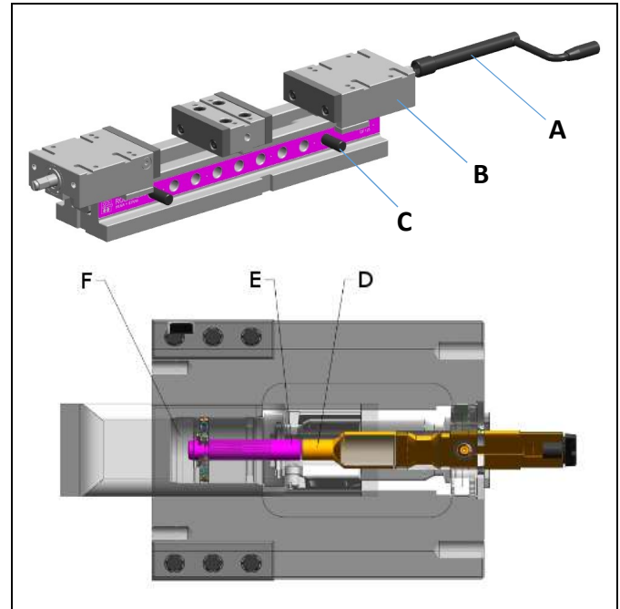
Abb. 1: Komponenten für Baureihe DF
