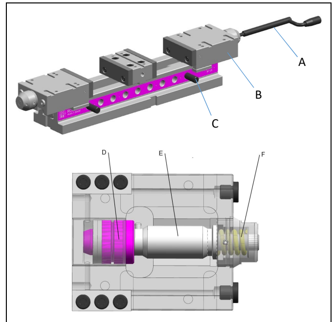
Abb. 1: Komponenten für Baureihe DF
