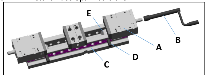
Abb. 4: Einstellen des Spannbereiches
