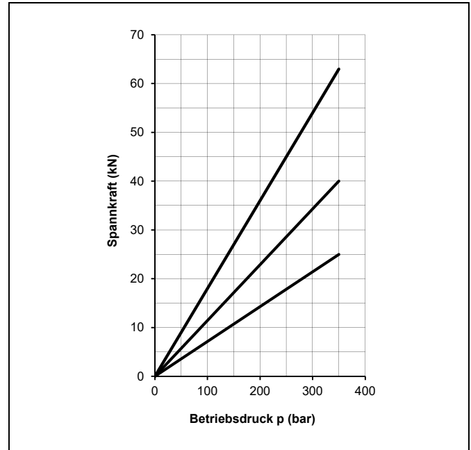
Abb. 9: Spannkraftverhältnisse
