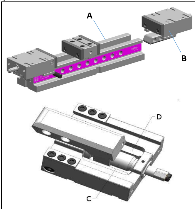
Abb. 8: Spannschlitten demontieren
