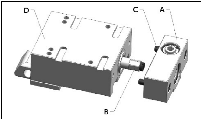
Abb. 7: Winkelantrieb
