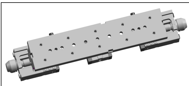
Abb. 3: Untersicht mit Befestigungs- und Positionsbohrungen
