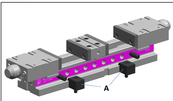
Abb. 2: Montagearten für Baureihe DF
