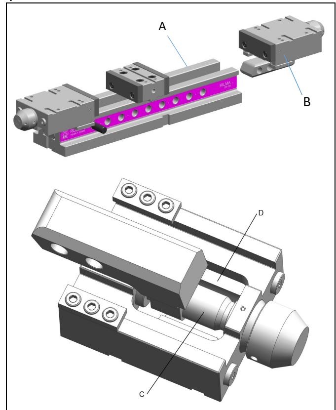
Abb. 8: Spannschlitten demontieren
