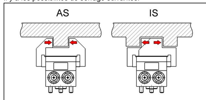
Fig. 2: Possibilités de serrage
