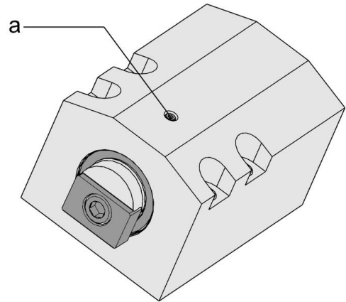
Abb. 5: Entlüftungsschraube
