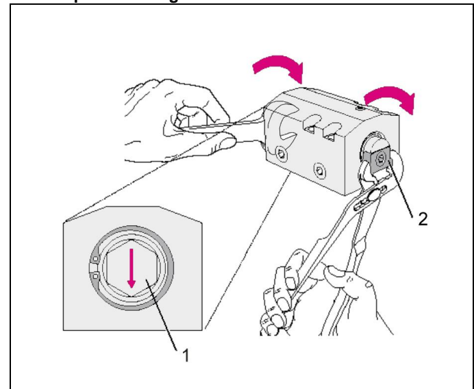
Abb. 2: Spannrichtung einstellen
