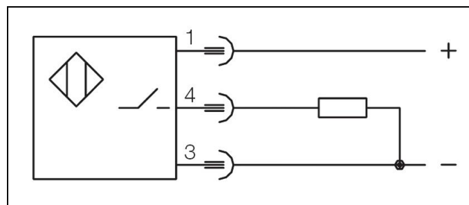
Fig. 9: Esquema eléctrico para pnp(+) sensor magnético
