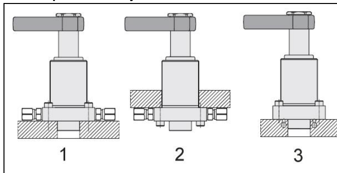
Fig. 3: Tipos de montaje
